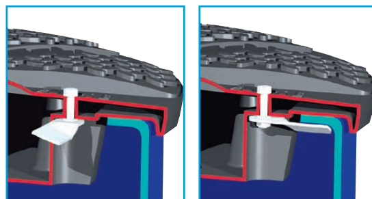
Detail van kinderveilig deksel van Varitanks
